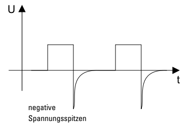
Impulsspannungen (an Zählspule)
